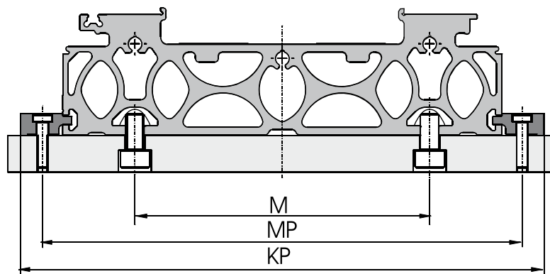
Maßtabelle - Befestigungsabstand HMR
