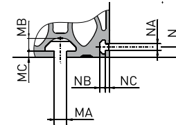
Ansicht X
