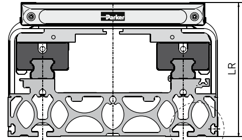
Trägerprofil „verstärkt“
