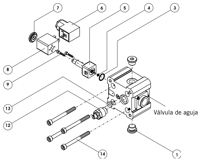
OSP-P40 / OSP-P50
